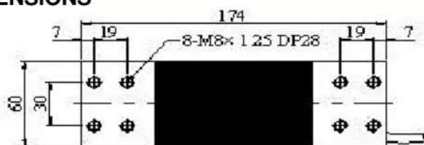
俯视图 (Top View)
