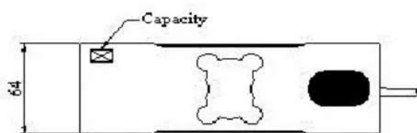
主视图 (Front View)
